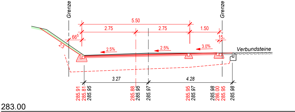
Querprofil 55 1'033.97
