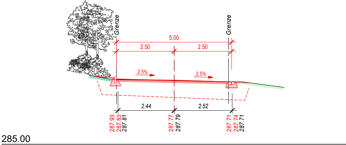
Querprofil 61 1'284.31
