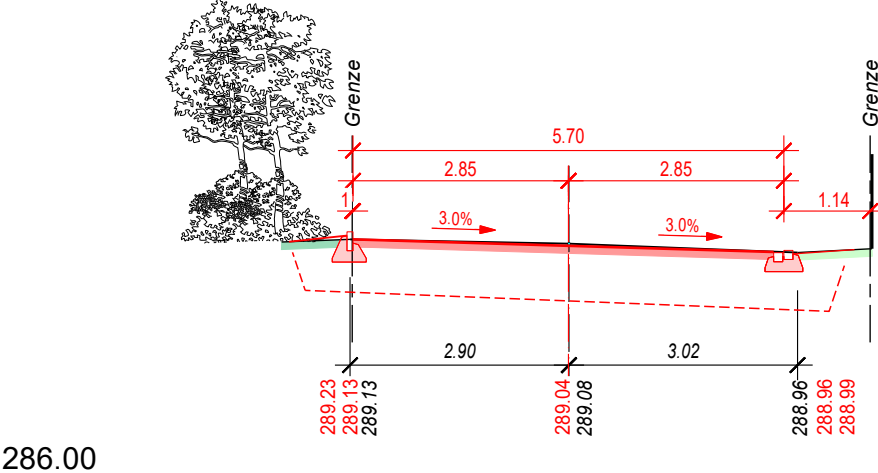
Querprofil 63 1'409.22
