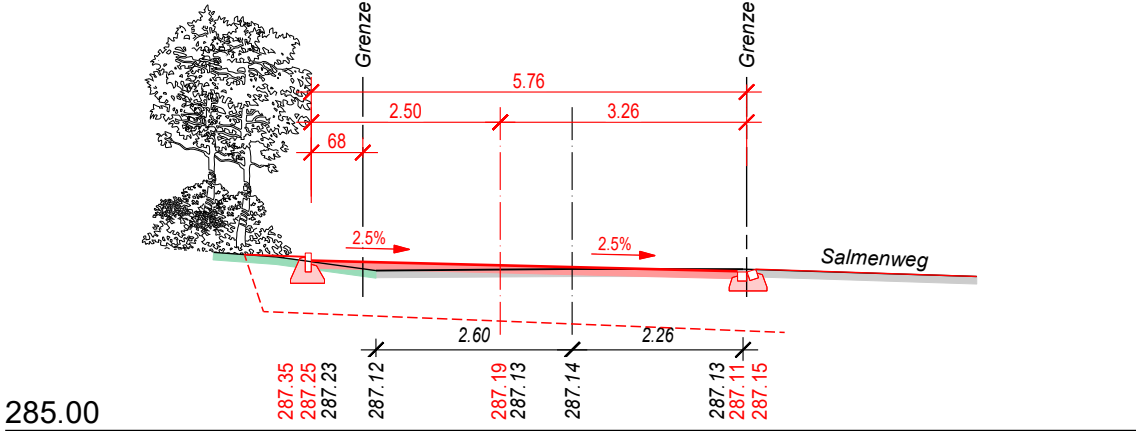
Querprofil 60 1'245.94
