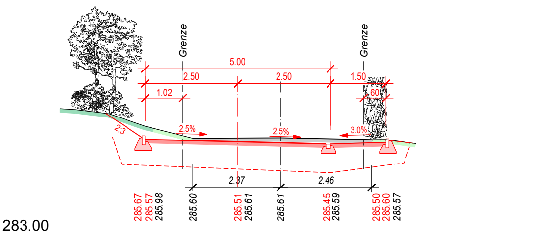
Querprofil 58 1'147.63
