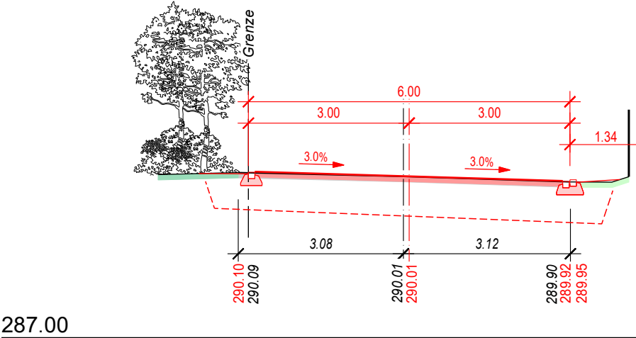
Querprofil 66 1'569.32
