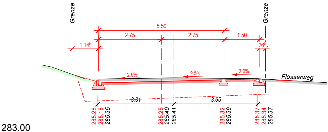
Querprofil 57 1'096.08
