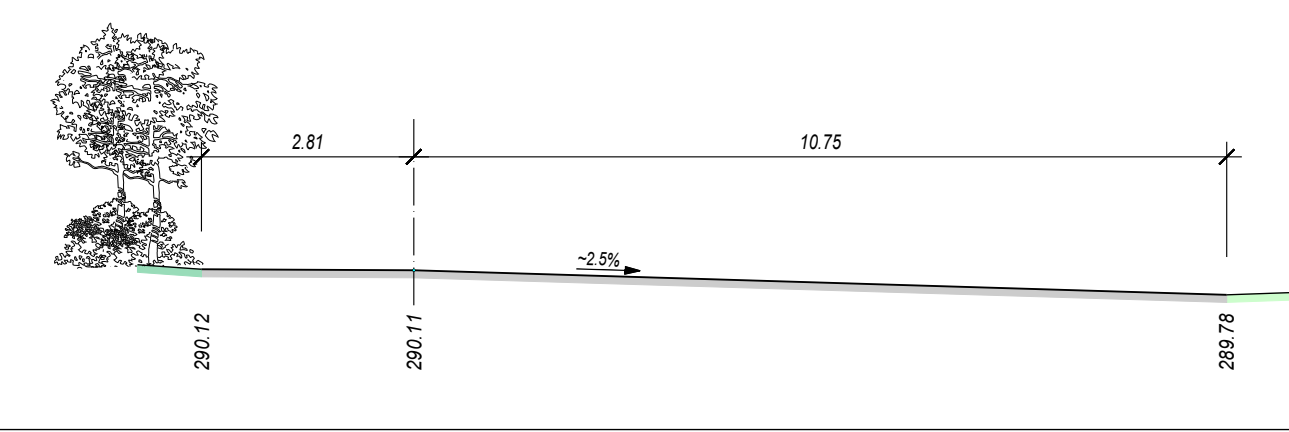
Querprofil 67 1'584.73
