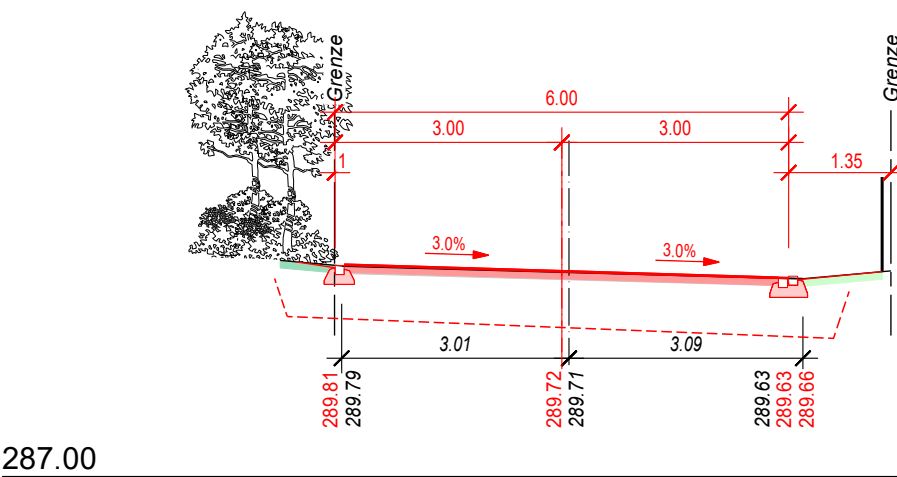
Querprofil 65 1'520.56
