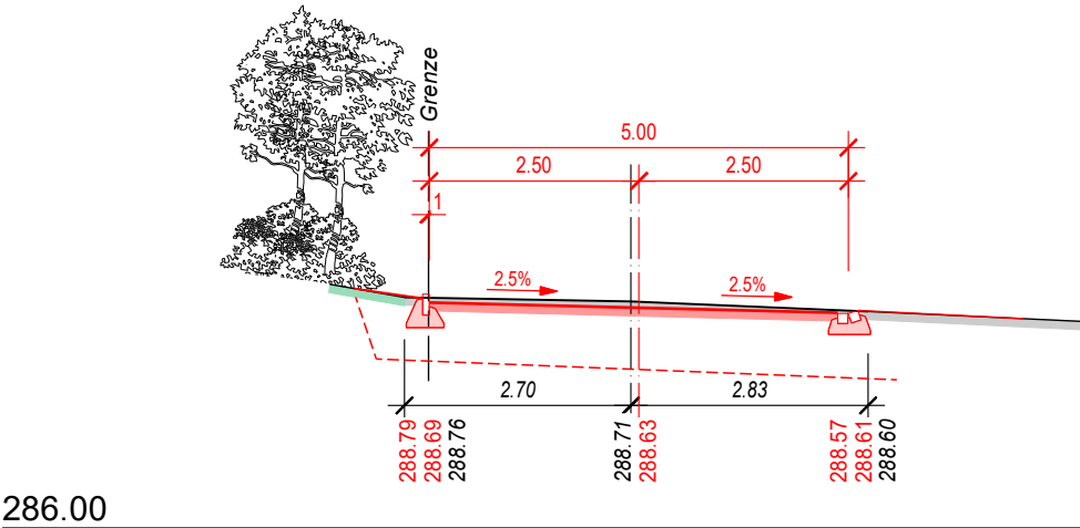
Querprofil 62 1'351.68
