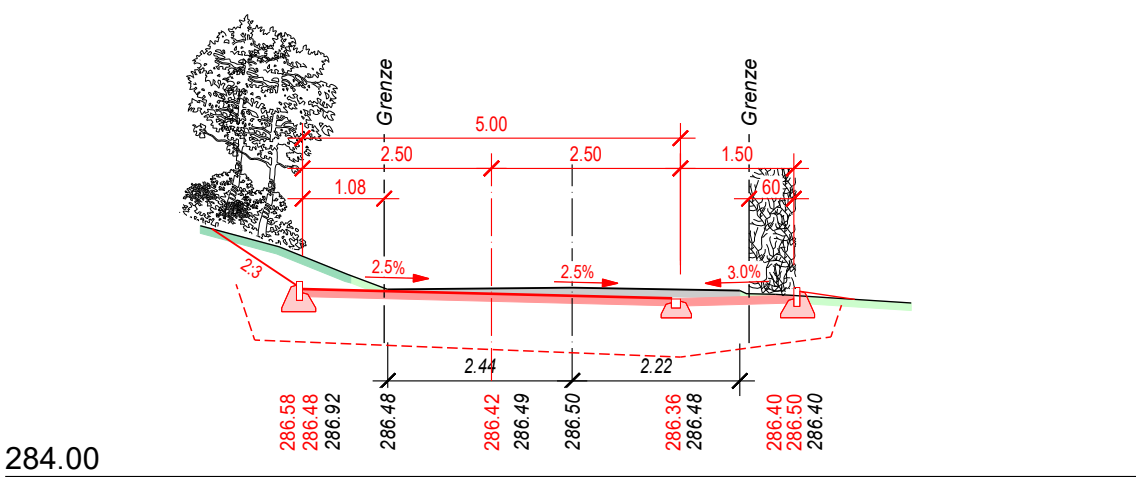
Querprofil 59 1'198.76
