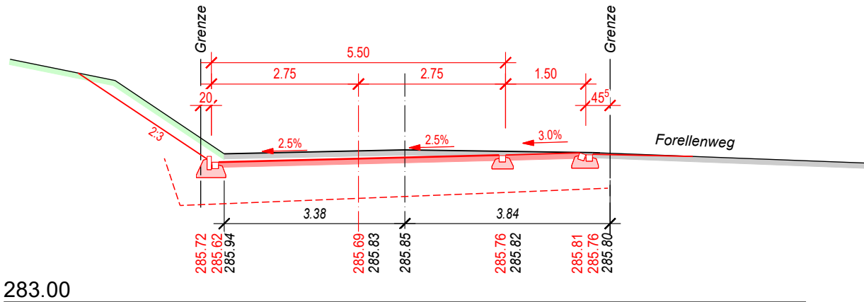
Querprofil 56 1'044.14
